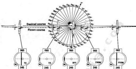
Figure 14. VOR Passage
