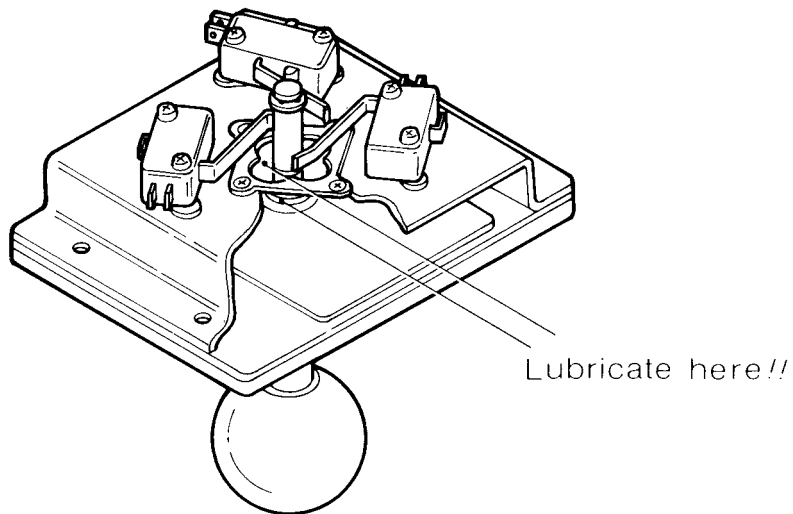
Fig. 5 Lubrication points
