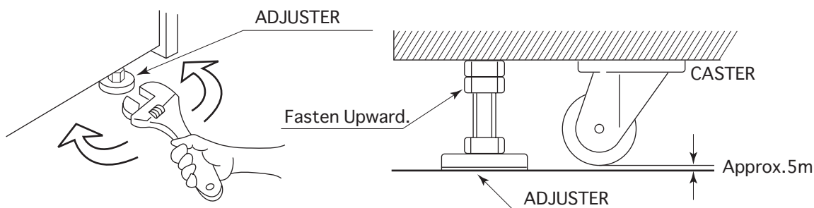
FIG. 6. 4 b ADJUSTER
